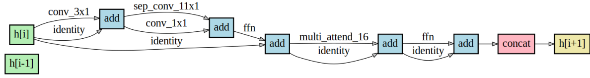
(a) NSGA-ViT
