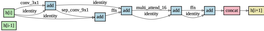
(a) NSGA-ViT
