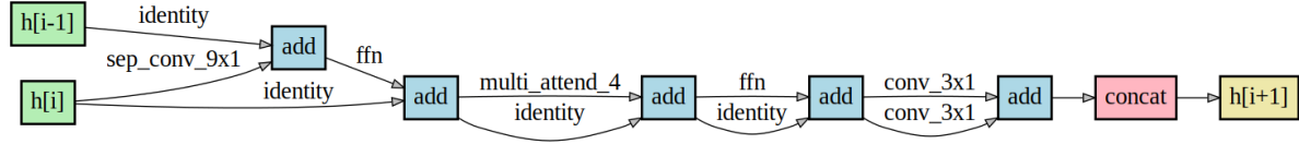
(b) NSGA-ViT-B
