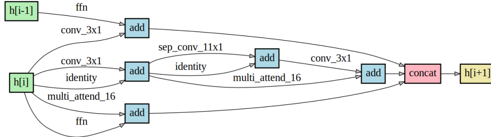
(d) NSGA-ViT-A
